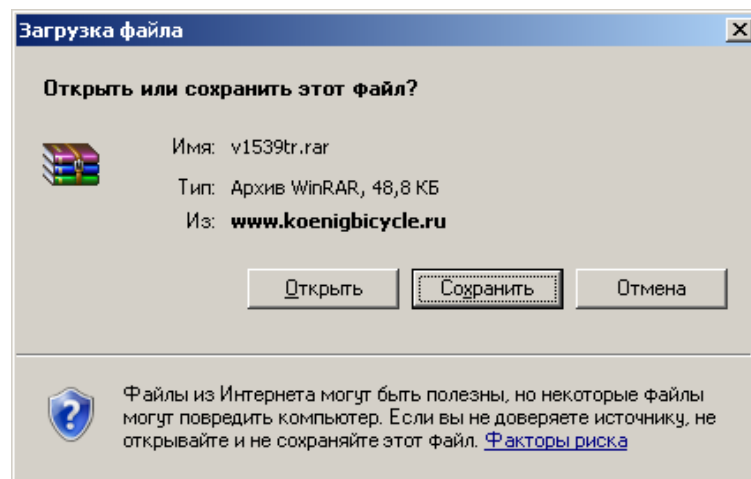
Рисунок 4. Сохранение трека.
